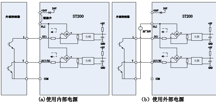
图 3-14 开路集电极 NPN 接线方式
