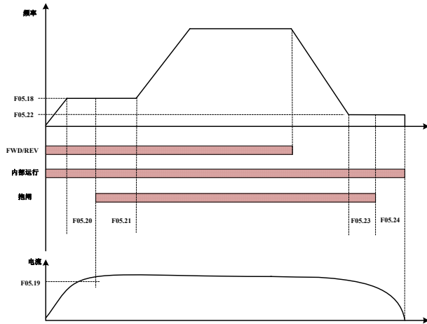
图 6-16 抱闸控制逻辑图
