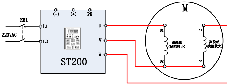
图 6-20 ST200 ( > 0.75\text{kW} ) 与单相电机正转接线图
