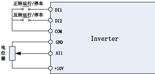
图 4 控制端子接线
