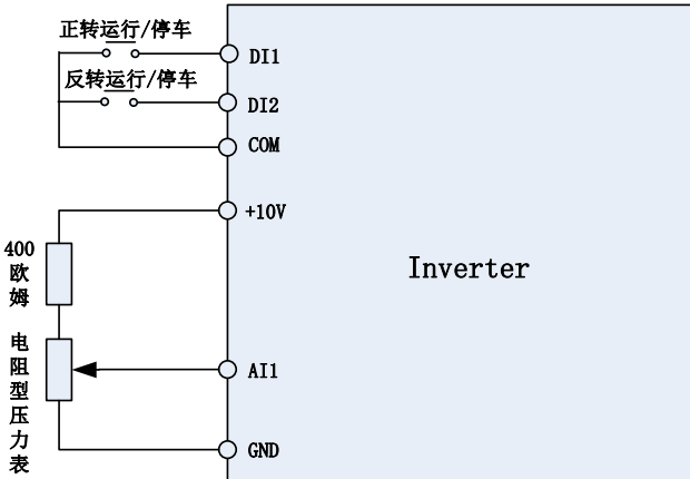
图 5 控制接线
