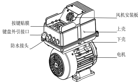
图 2-3 0.75~2.2kW 外形图
