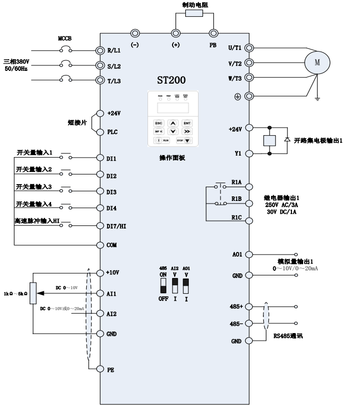
图 3-9 ST200 变频器接线示意图
