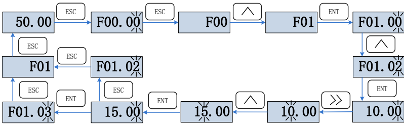
图 4-3 三级菜单操作举例
