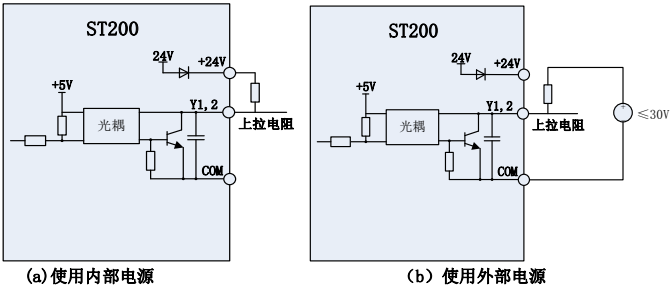
图 3-16 端子接上拉电阻输出时的接线方式
