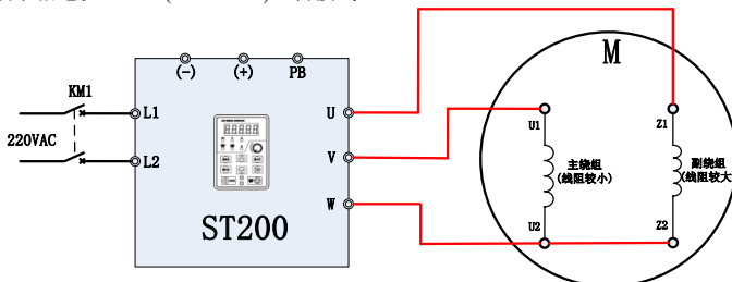
图 6-18 ST200 (≤0.75kW) 与单相电机正转接线图
