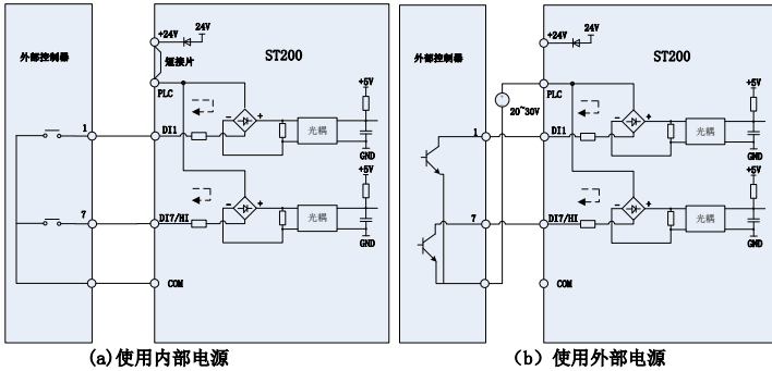
图 3-13 干接点方式
