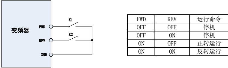
图 6-9 两线模式 2 控制示意图
