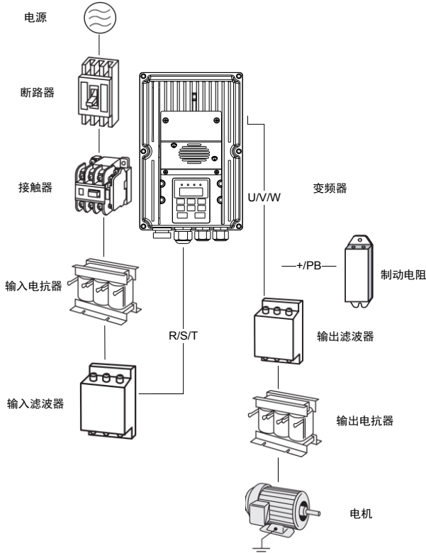
图 3-8 产品外围器件及配线
