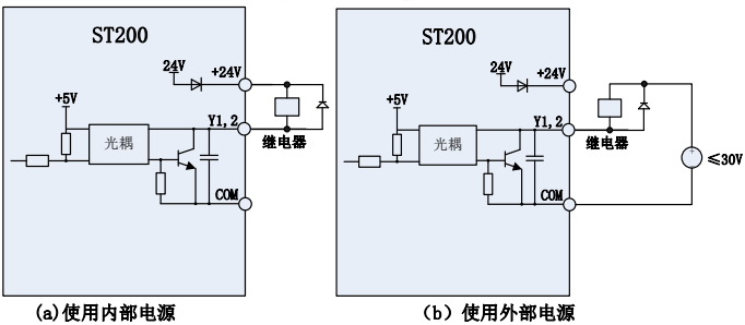
图 3-17 端子驱动继电器时的接线方式
