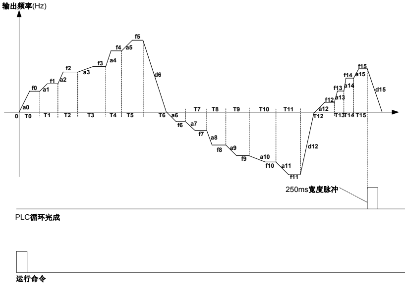
图 6-30 PLC 单循环后停机示意图
