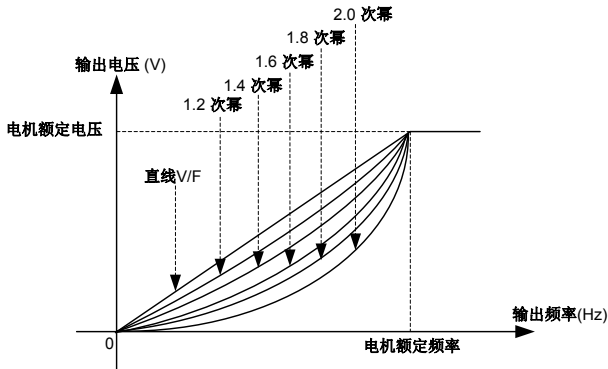
图 6-24 VF 曲线示意图
