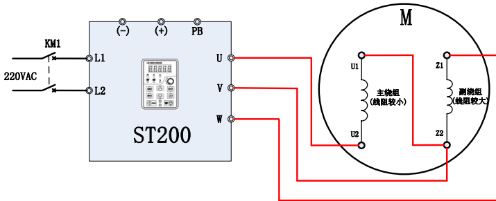
图 6-21 ST200 ( > 0.75\text{kW} ) 与单相电机反转接线图
