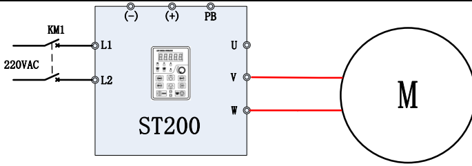
图 6-22 ST200( \leq 0.75\text{kW} )与单相电机接线图
