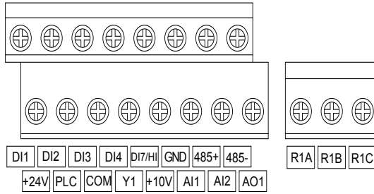
图 3-11 控制端子示意图
