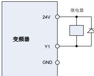
图 6-13 Y1 控制外部继电器示意图
