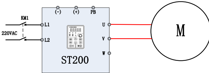
图 6-23 ST200 ( > 0.75\text{kW} ) 与单相电机接线图
