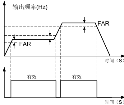
图 6-14 FAR 功能示意图
