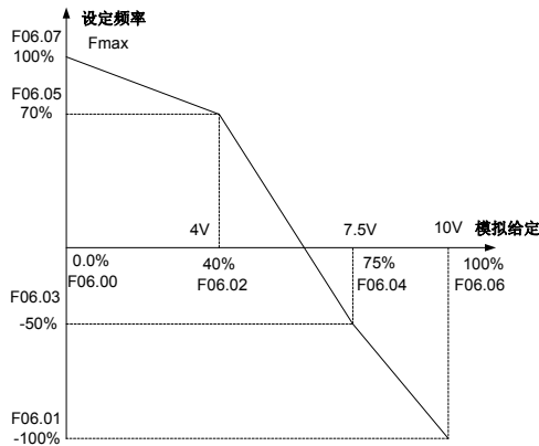
图 6-17 (2) 代码参数设定示意图
