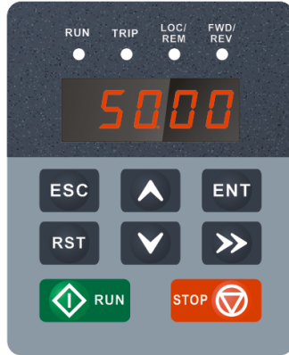
图 4-1 操作面板示意图
