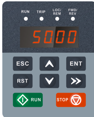
图 8 操作面板示意图
