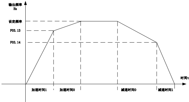
图 6-7 加减速时间切换频率示意图
