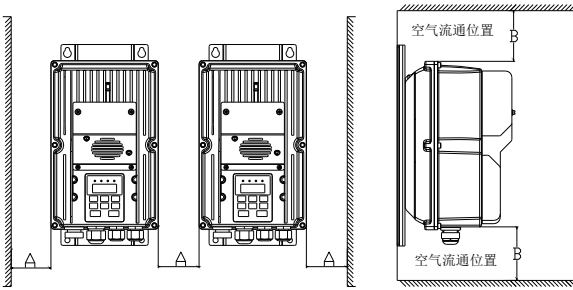
图 3-3 多台变频器并排安装方向及空间
