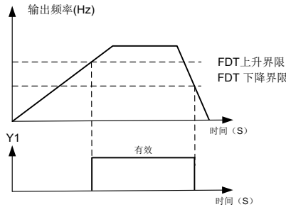
图 6-15 FDT 功能示意图
