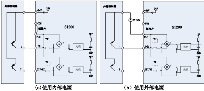
图 3-15 开路集电极 PNP 接线方式
