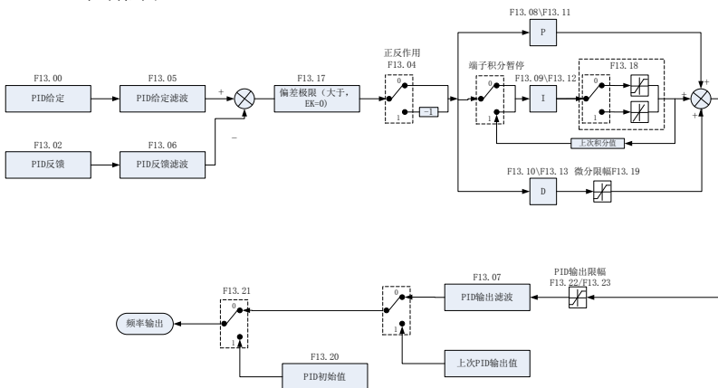
图 6-33 PID 控制框图
