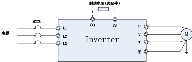
图 2 主回路接线
