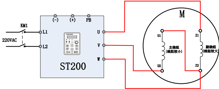
图 6-19ST200 ( \leq 0.75\text{kW} ) 与单相电机反转接线图
