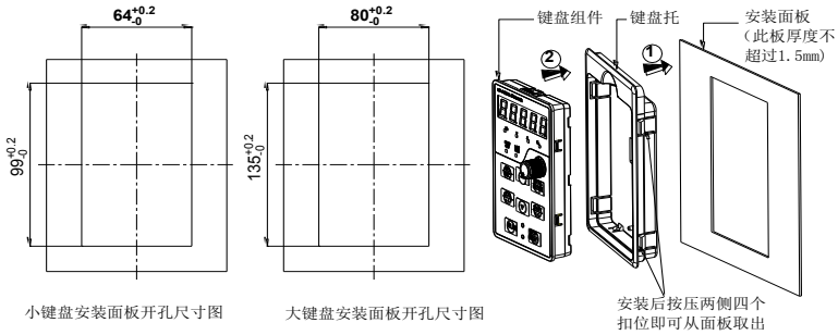
图 2-7 键盘外置安装开孔尺寸图
