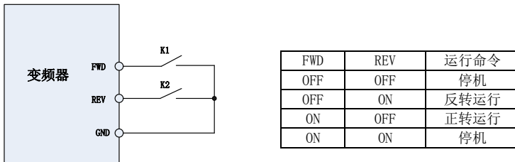
图 6-8 两线模式 1 控制示意图
