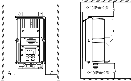
图 3-2 单台变频器安装方向及空间
