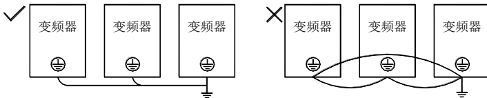
图 3-18 变频器接地处理
