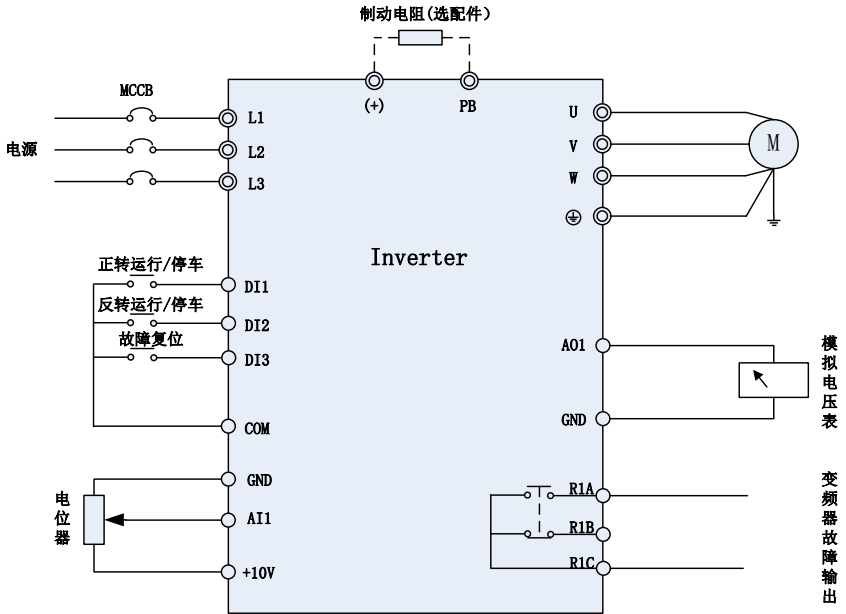
图 6 整体接线
