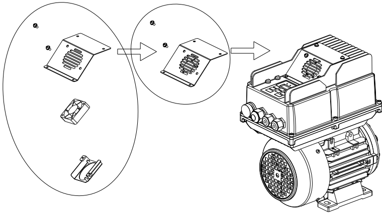
图 8-2 (a) 安装风扇引线图
