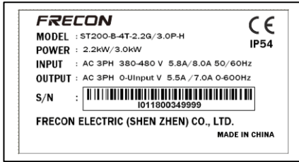
图 2-1 产品铭牌
