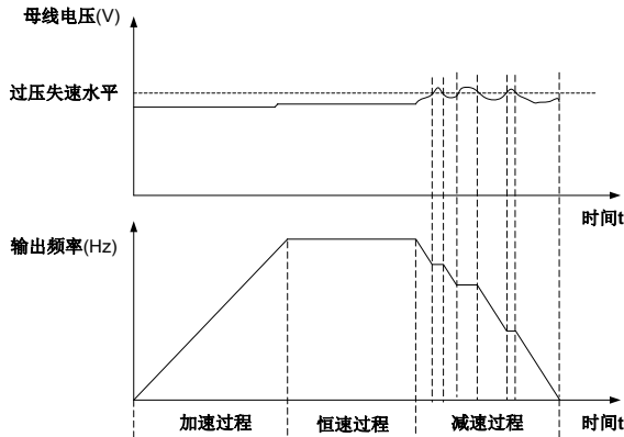
图 6-28 过压失速模式 1 示意图
