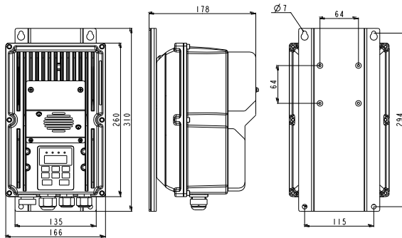
图 2-5 0.75~2.2kW 壁挂安装示意图
