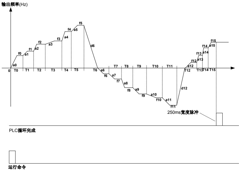
图 6-31 PLC 单循环后保持最终值示意图
