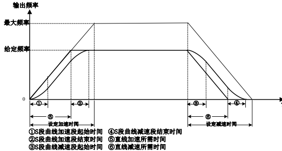
图 6-6 S 曲线加减速示意图
