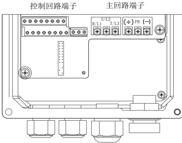
图 3-10 0.75~2.2kW 主回路端子示意图
