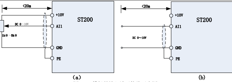
图 3-12 模拟量输入端子接线示意图
