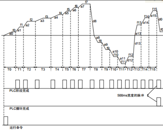
图 6-32 PLC 连续循环示意图
